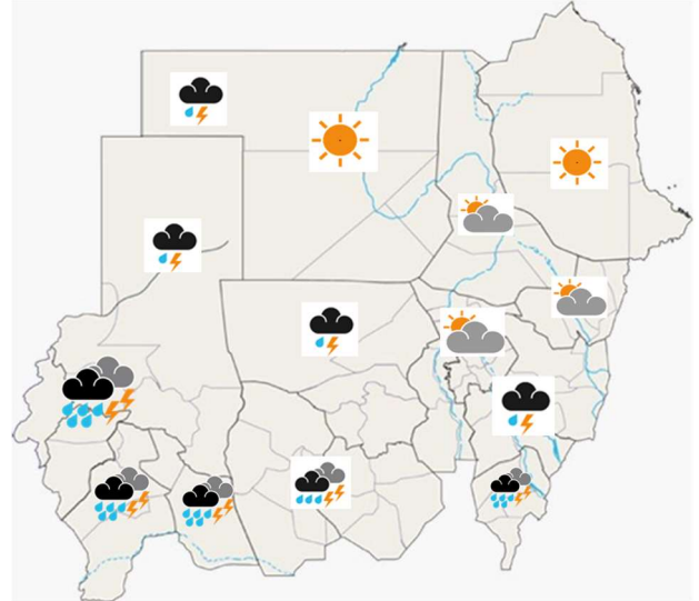
خريطة توقعات الطقس المتوقعة ليوم الاحد ٣١ اغسطس ٢٠٢٥
