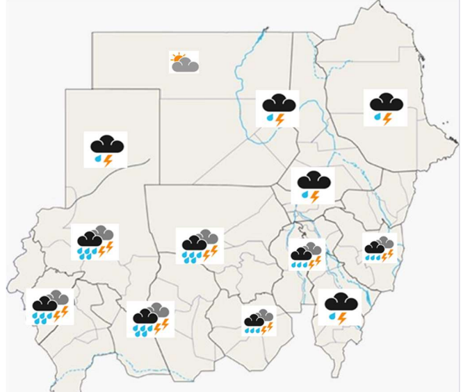
خريطة توقعات الطقس المتوقعة ليوم الجمعة ١٥ أغسطس ٢٠٢٥
